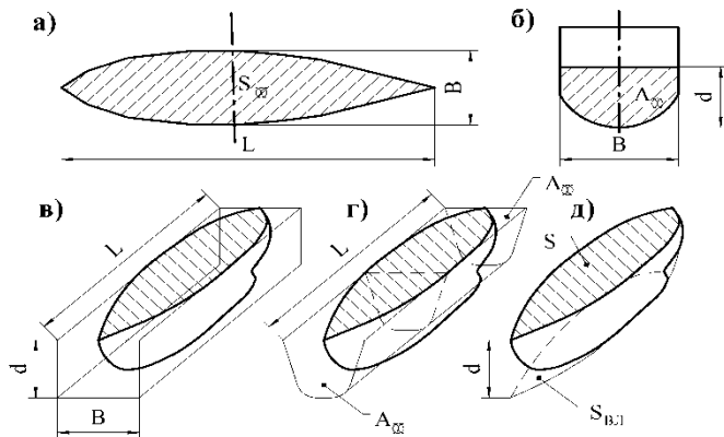
Рис.7. – Коэффициенты полноты
