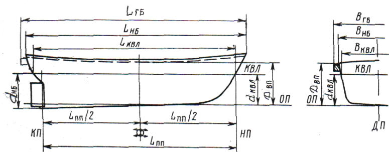
Рис.6. Главные наибольшие и габаритные размеры судна
