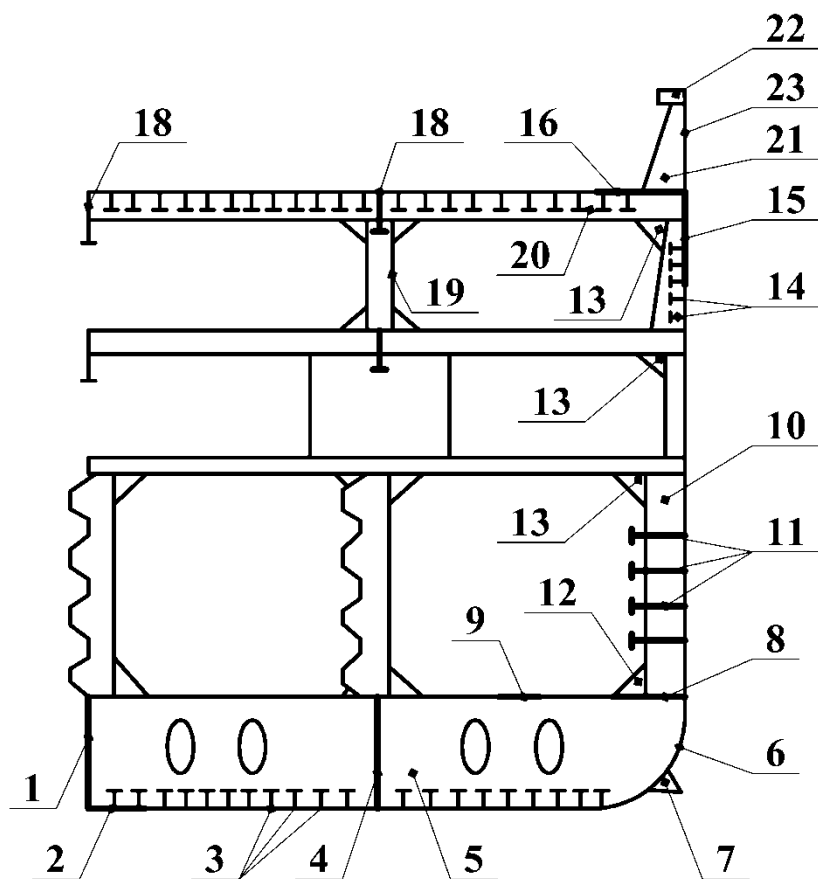
Рис. 4. Конструктивный мидель-шпангоут
